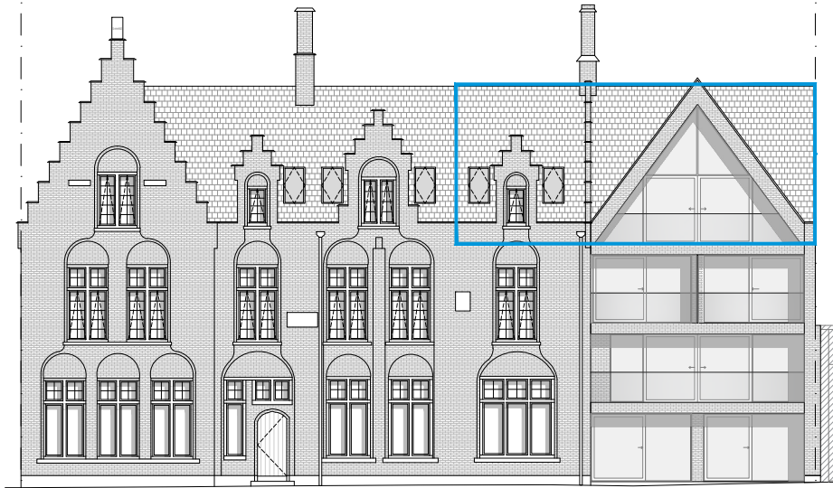
Voorgevel
